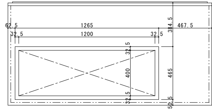
A 矢视图(底面詳細図)
