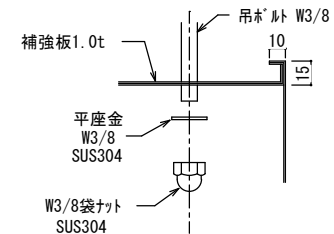
Y部 詳細図
