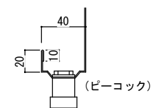
Z部 詳細図
