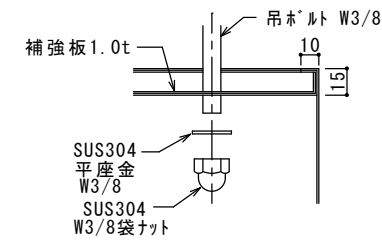
Y部 詳細図
